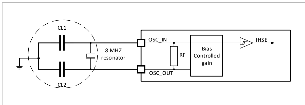
图 18. 使用 8 MHz 晶体的典型应用
