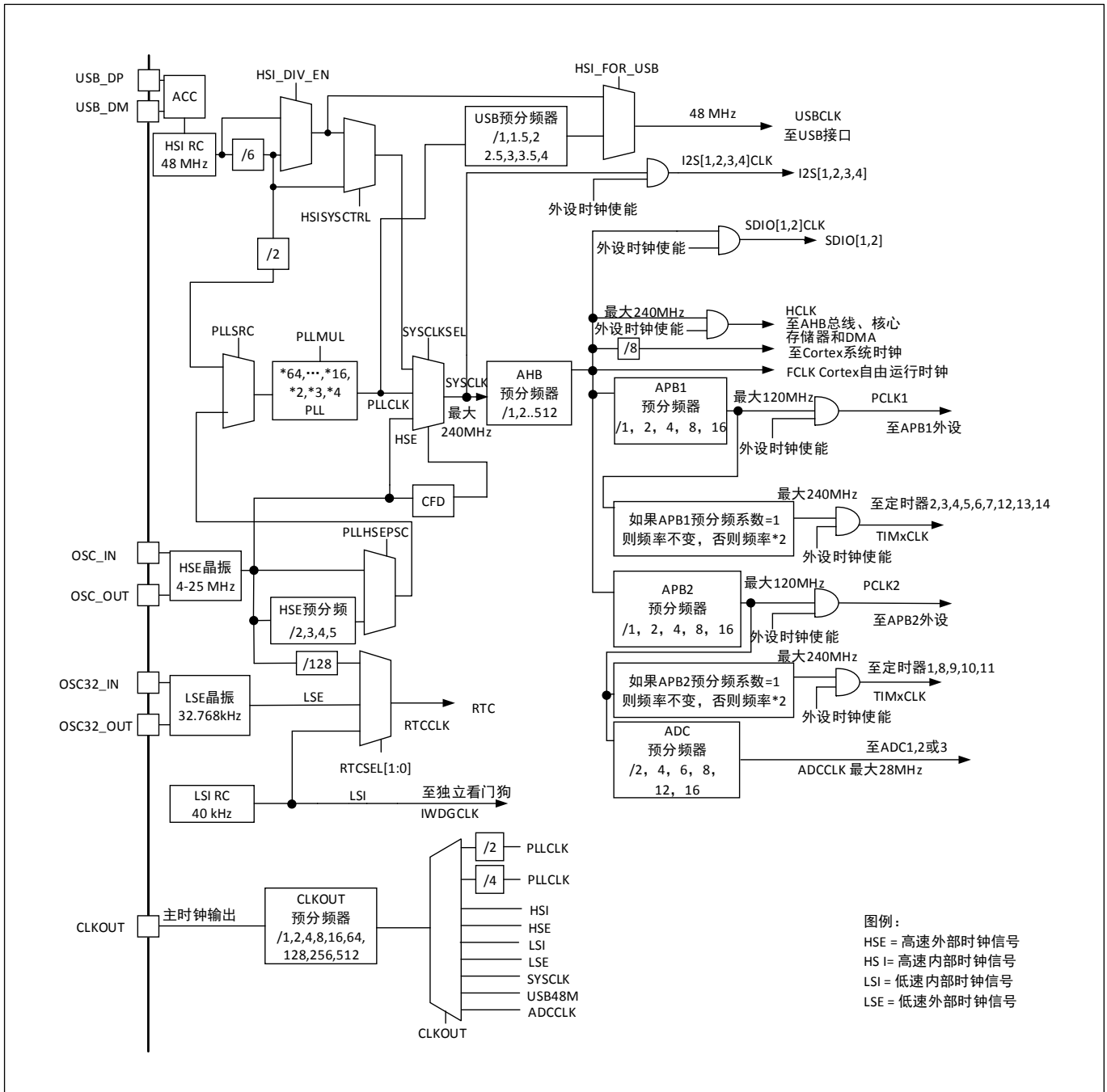
图 2. 时钟树
