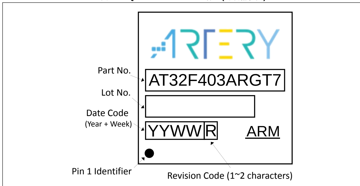
图 47. LQFP64 – 10 x 10 mm 标记(封装俯视图)
