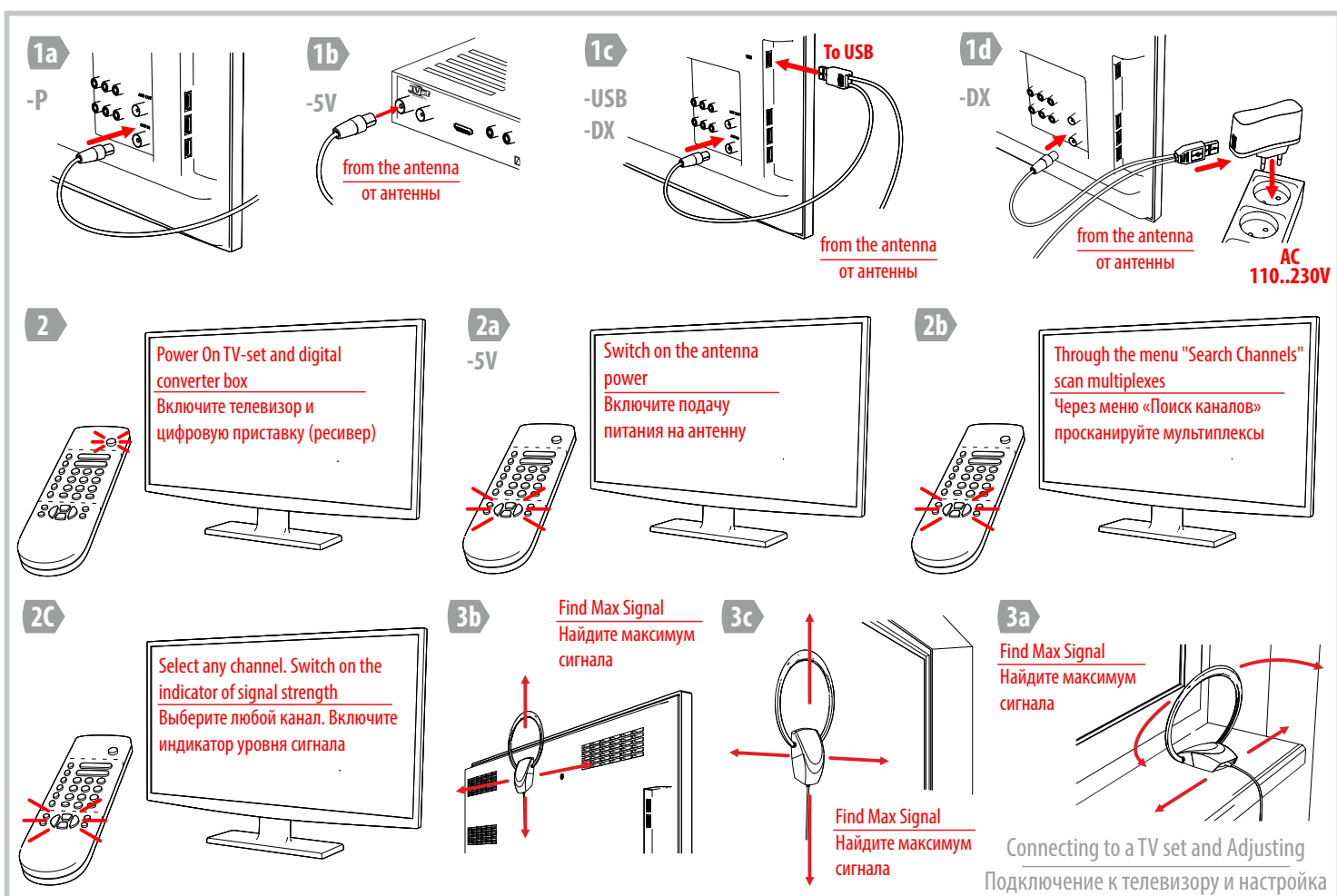
Installing on a window glass Установка на оконное стекло
