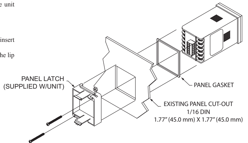
1/16 DIN Installation
