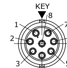
WIRING END W6280-8SG-P-5XX
