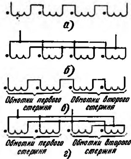
Рис 2 8. Электрические схемы последовательного и параллельного соединений вторичных обмоток трансформаторов типа ТПП: а — броневой конструкции; б — стержневой конструкции.
