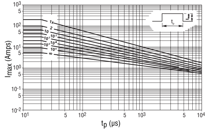
Model Size 1206 - (AV 14 K 1206 201 ~ AV 40 K 1206 201)
