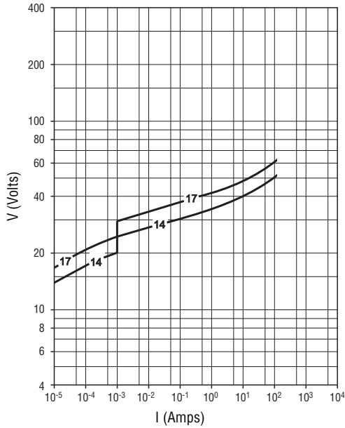
Model Size 0805 - (AV 14 K 0805 121 ~ AV 17 K 0805 121)
