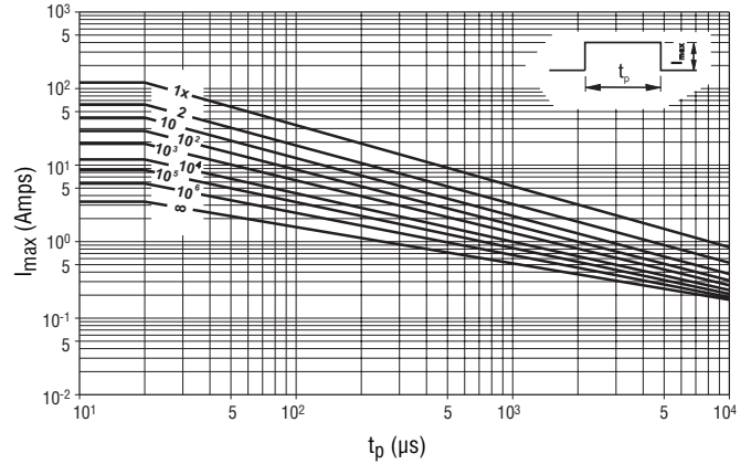
Model Size 0805 - (AV 14 K 0805 121 ~ AV 17 K 0805 121)
