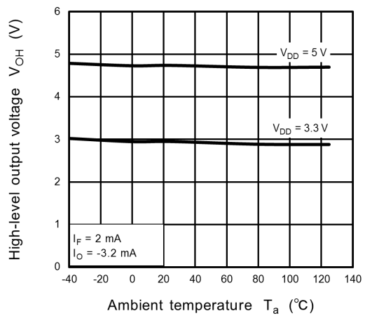
Fig. 13.2.6 V_{OH} - T_a
