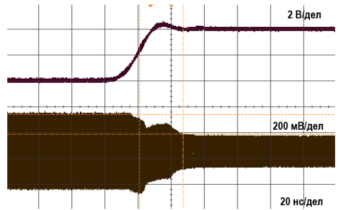
Время включения
