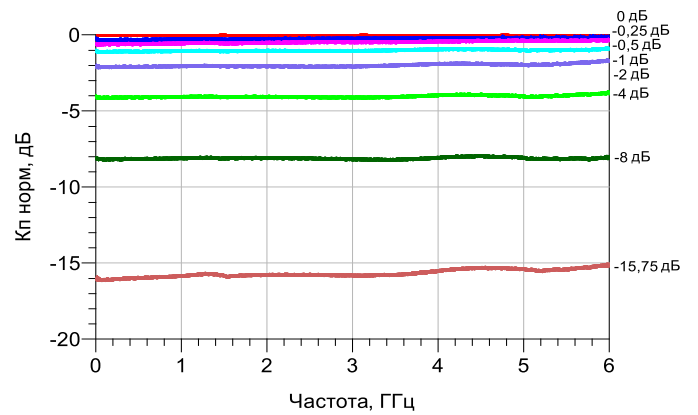
Зависимость нормированного коэффициента ослабления от частоты сигнала
