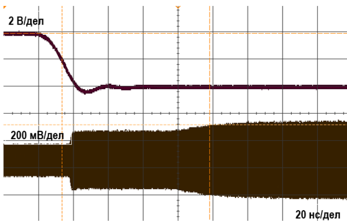
Время выключения
