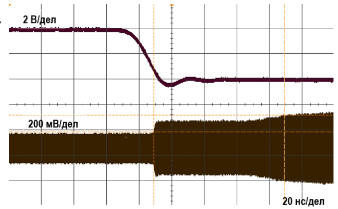
Время включения
