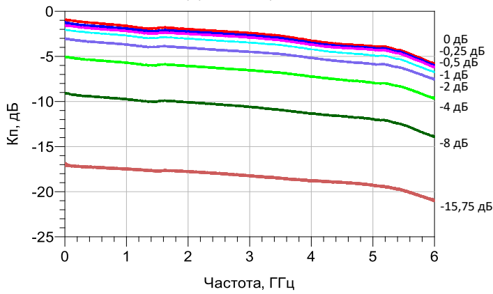
Зависимость коэффициента передачи от частоты сигнала
