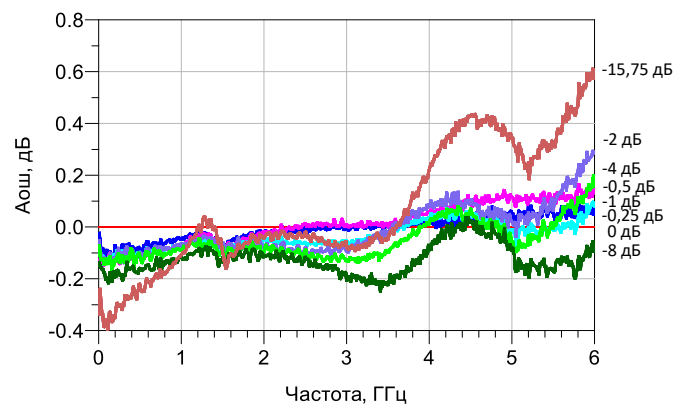
Зависимость амплитудной ошибки от частоты сигнала
