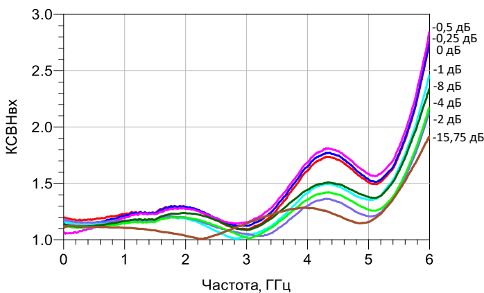
Зависимость КСВН на входе от частоты сигнала
