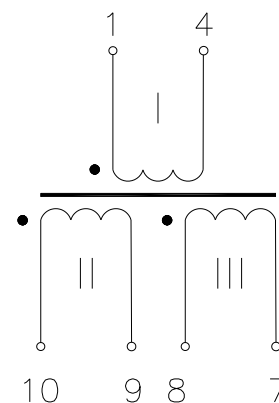
Схема электрическая
