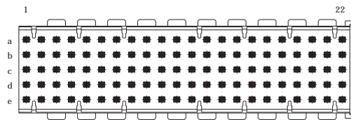
Bestückungsplan - contact layout
