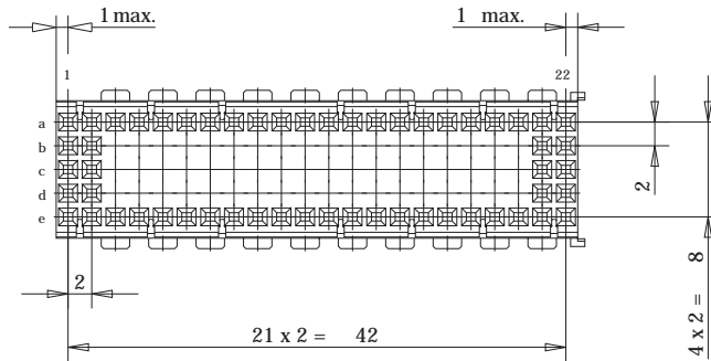
Bestückungsplan - contact layout
