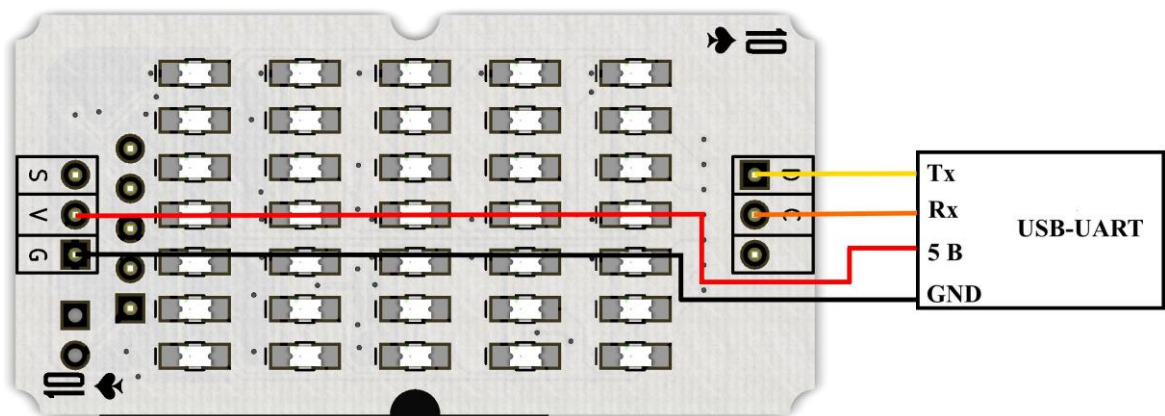
Питание модуля от переходника USB-UART
