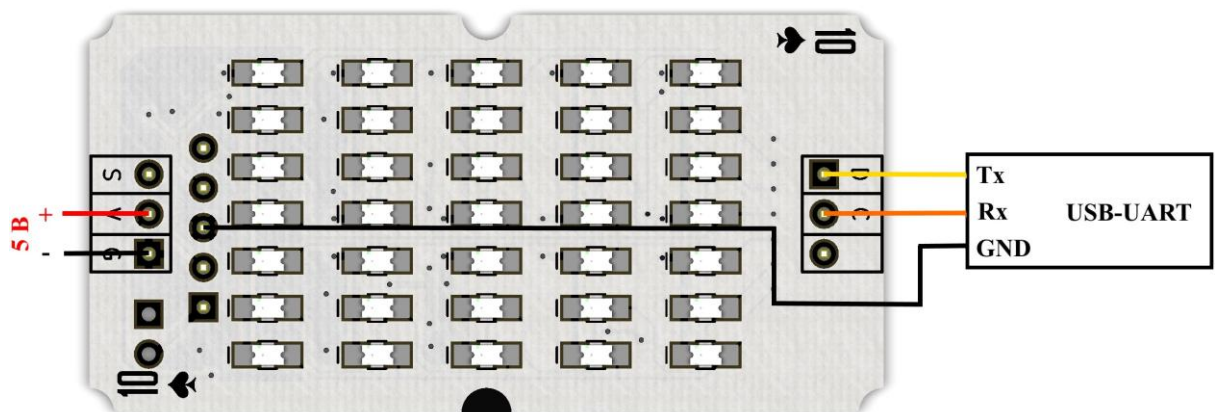
Питание модуля от источника 5 В
