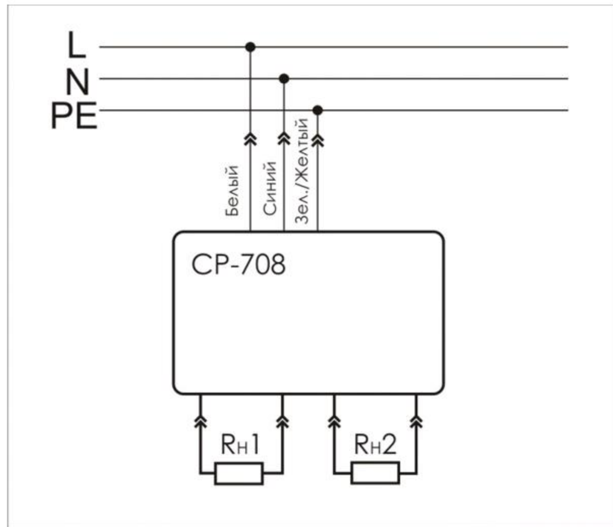
Схема подключения CP-708
