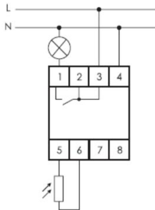
Схема подключения
