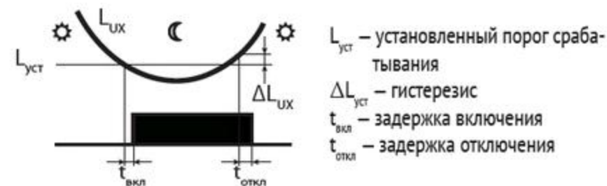
Диаграмма работы фотореле
