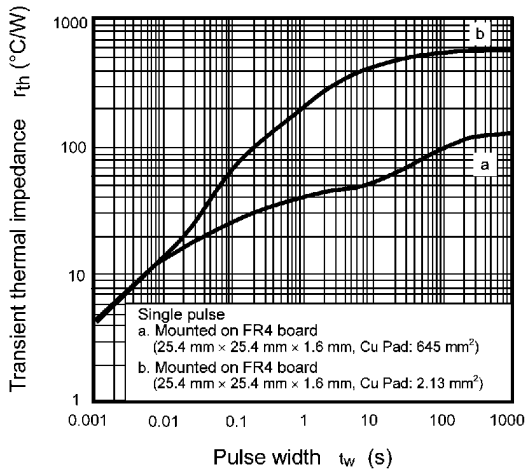
Fig. 7.13 r_{th} - t_w
