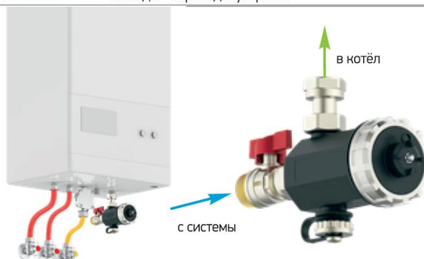
Схема 1 Расположение корпуса – фронтальное. Выходы - перпендикулярные.
