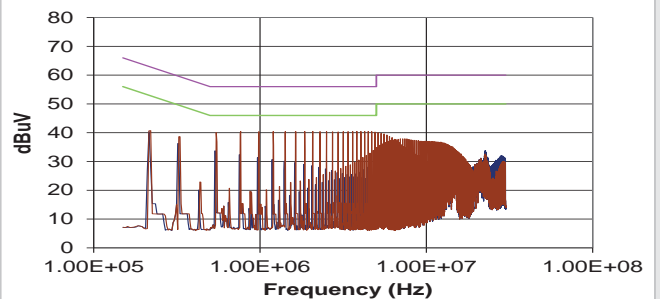
MGJ1D121503MPC
