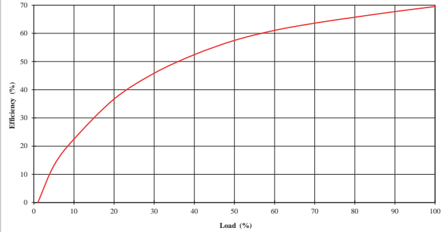
MGJ1D151505MPC
