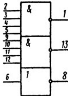
Условное графическое обозначение К176ЛП12
