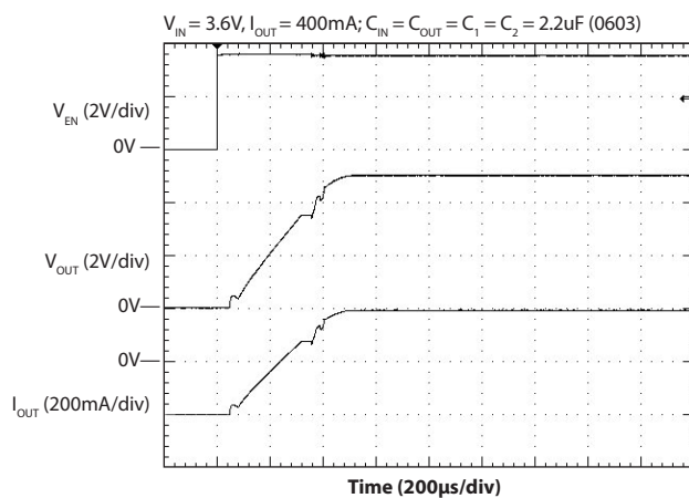
Startup (400mA)
