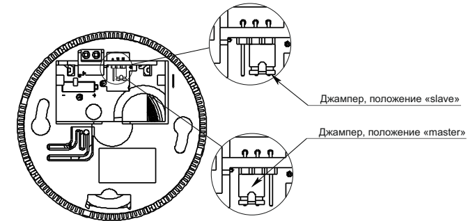
Рисунок А2 – Положения джампера
