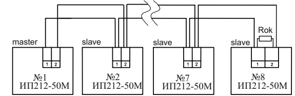
Рисунок А1 – Схема объединения извещателей в шлейф
