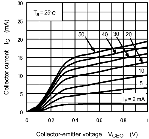
Fig. 11.8 I_C - V_{CEO}
