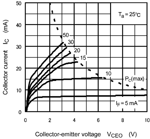
Fig. 11.7 I_C - V_{CEO}
