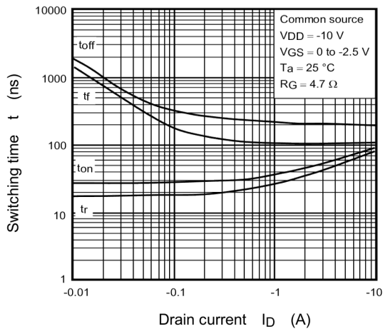
Fig. 7.11 t - I_D
