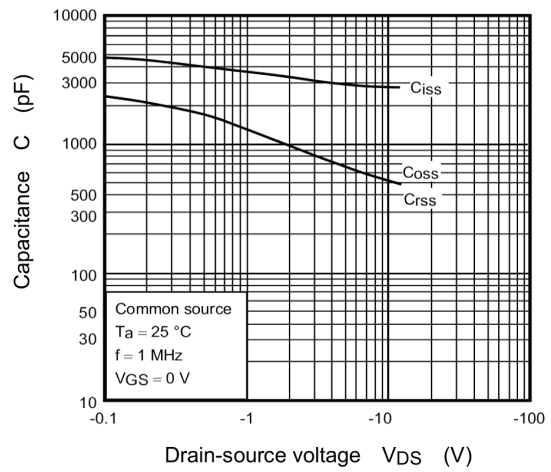
Fig. 7.10 C - V_{DS}
