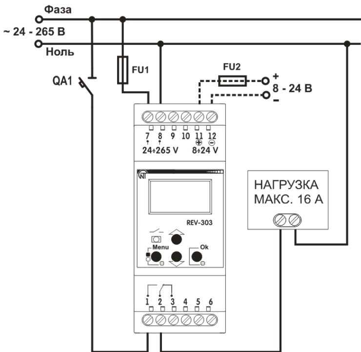
QA1 - Автоматический выключатель (макс. 16 А); FU1, FU2 - Плавкий предохранитель (макс. 1 А).
