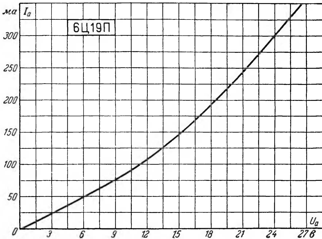
Анодная характеристика лампы 6Ц19П.
