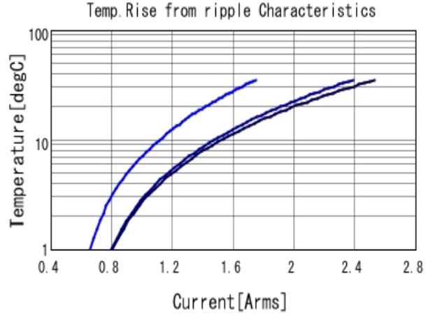
■ GCM21BR71H224KA37 Temp. rise ■ 300kHz ■ 600kHz ■ 1MHz
