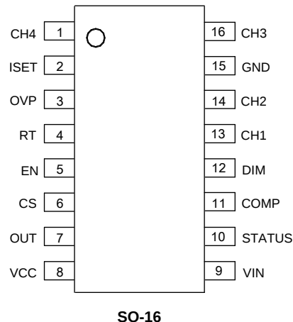
SO-16
