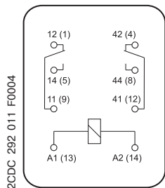
CR-M с 2 переключающими контактами
