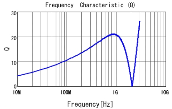
■ LQG15HS27NJ02 Q
