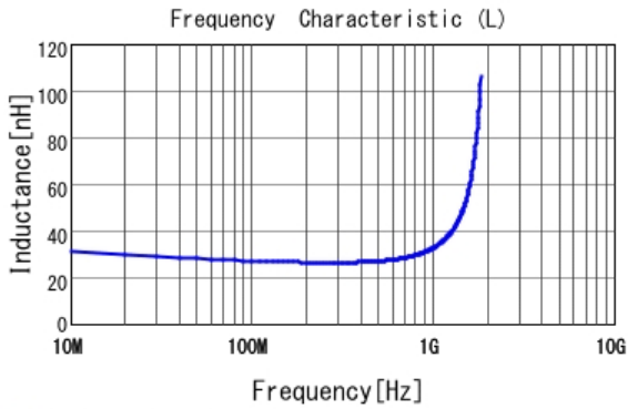
■ LQG15HS27NJ02 L
