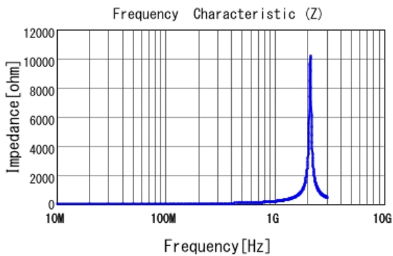
■ LQG15HS27NJ02 |Z|
