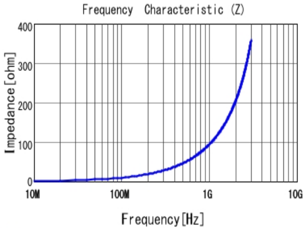
■ LQW15AN15NH00 |Z|
