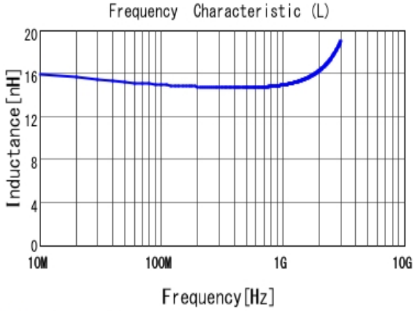
■ LQW15AN15NH00 L
