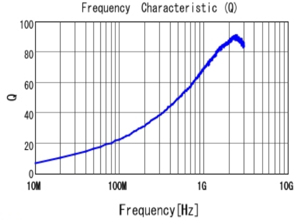
■ LQW15AN15NH00 Q
