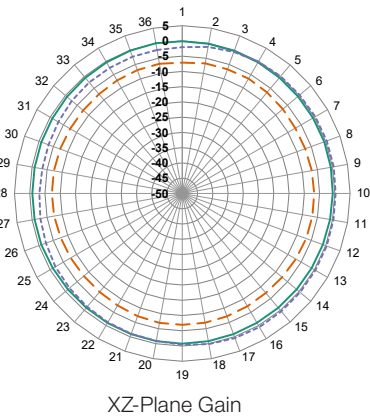
XZ-Plane Gain
