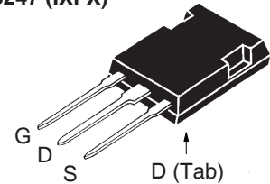
PLUS247 (IXFX)
