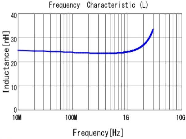
■ LQW15AN24NJ00 L
