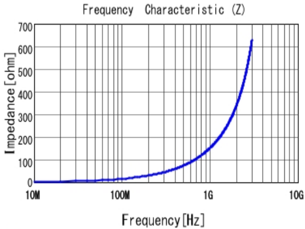
■ LQW15AN24NJ00 |Z|
