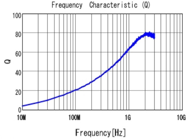
■ LQW15AN24NJ00 Q
