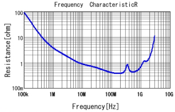
■ GA342QR7GD681KW01 R DCOV, 25degC
