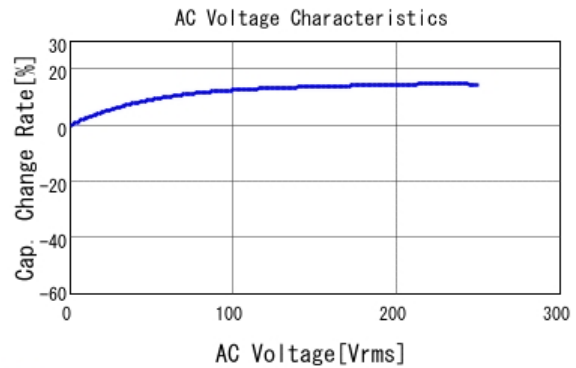
■ GA342QR7GD681KW01 C-AC Voltage capchange, DCOV, 25.0d
