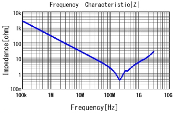
■ GA342QR7GD681KW01 |Z| DCOV, 25degC
