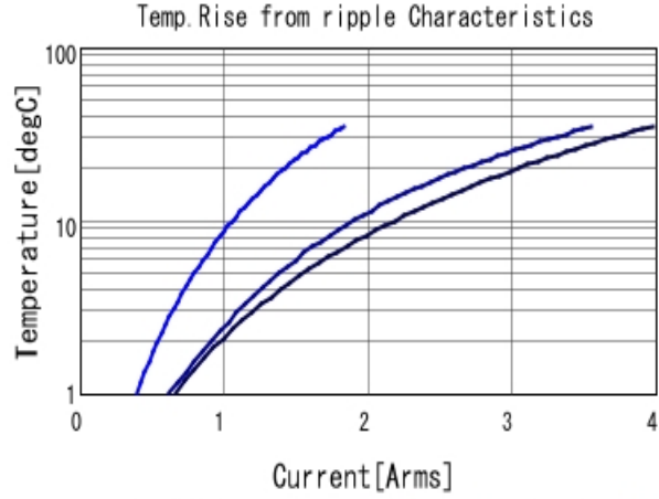
GCM31MR71H105KA55 Temp. rise ■ 100kHz ■ 500kHz ■ 1MHz
