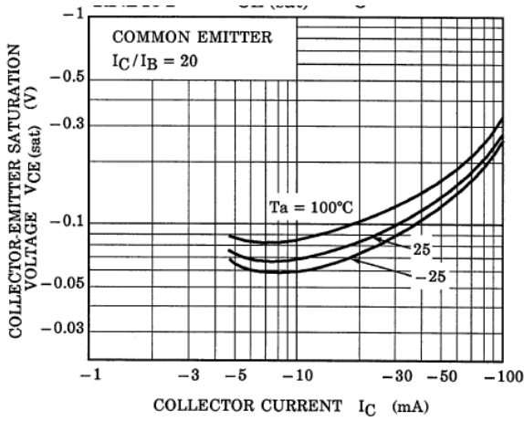
Fig. 10.19 RN2401 V_{CE(sat)}-I_C
