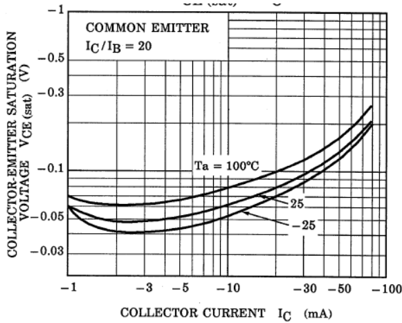
Fig. 10.21 RN2403 V_{CE(sat)}-I_C
