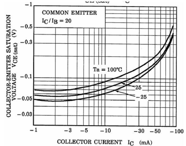
Fig. 10.24 RN2406 V_{CE(sat)}-I_C
