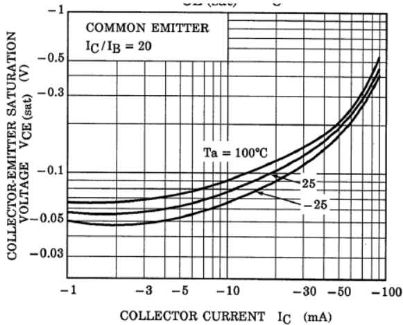
Fig. 10.23 RN2405 V_{CE(sat)}-I_C
