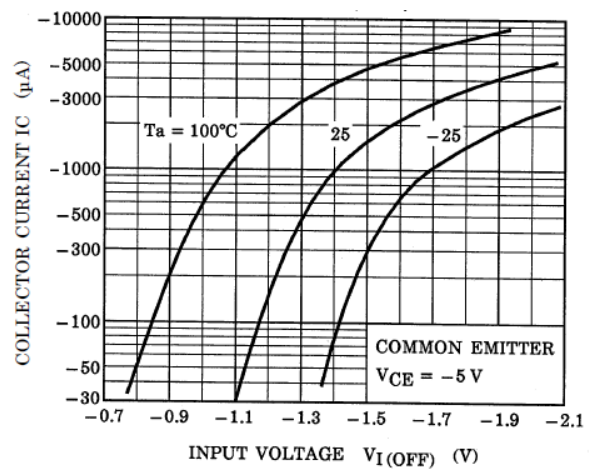
Fig. 10.10 RN2404 I_C - V_{I(OFF)}
