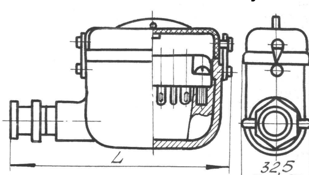
Розетка РП14А кабельная угловая
