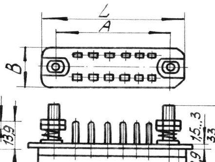
Розетка РП14 с ловителями вариант II
