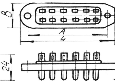
Вилка РП14 с ловителями облегченная
