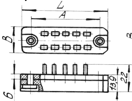
Розетка РП14 с ловителями облегченная вариант II
