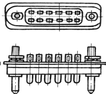
Вилка РП14 с ловителями (вариант)
