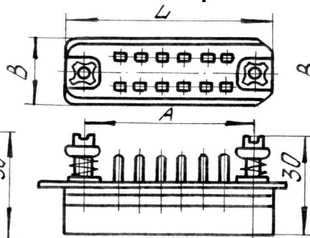
Розетка РП14 с ловителями вариант I
