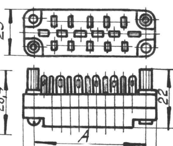
Розетка РП14А
