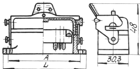
Вилка кабельная прямая РП14А
