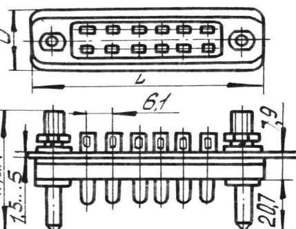
Вилка РП14 с ловителями
