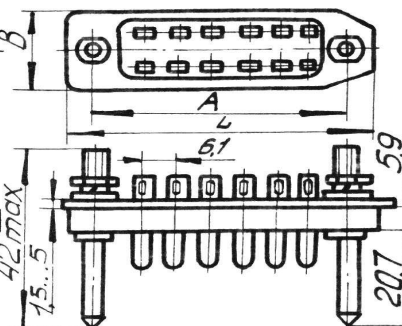
Вилка РП14 с ловителями (вариант)
