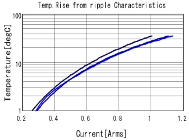
GJM1555C1H100JB01 Temp. rise 700MHz 1GHz 2GHz
