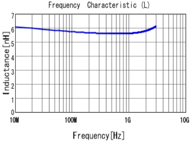
■ LQW15AN5N8B00 L
