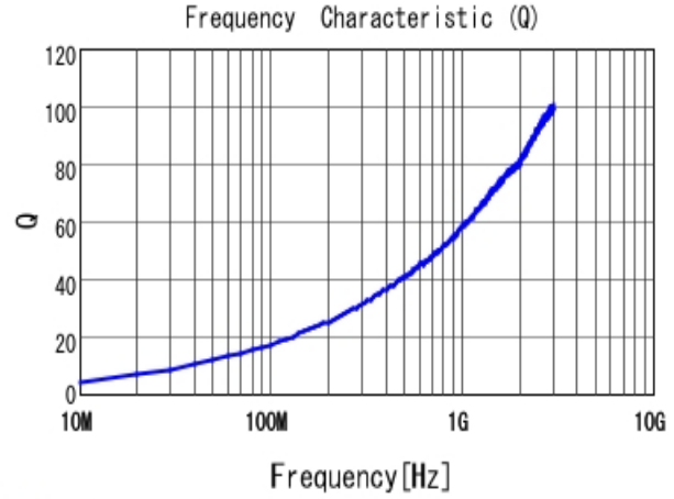
■ LQW15AN5N8B00 Q
