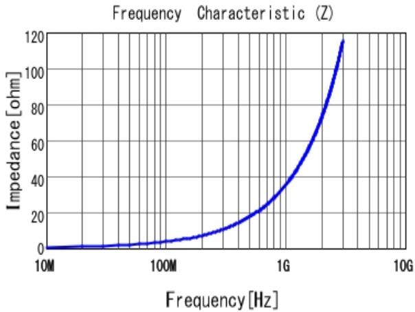
■ LQW15AN5N8B00 |Z|
