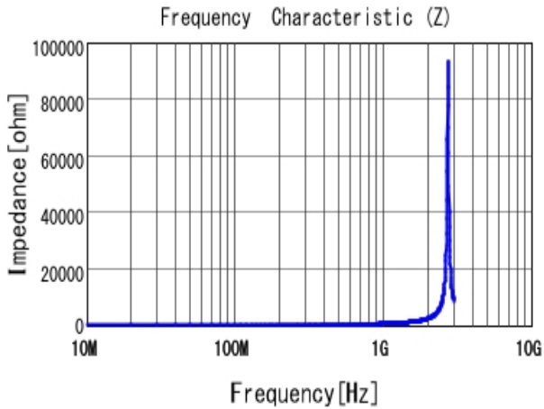
■ LQW15AN91NG00 |Z|
