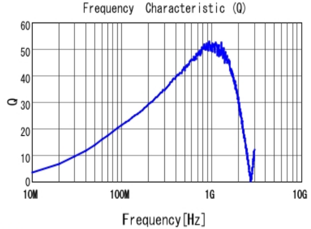
■ LQW15AN91NG00 Q
