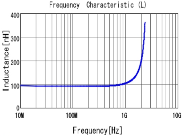
■ LQW15AN91NG00 L
