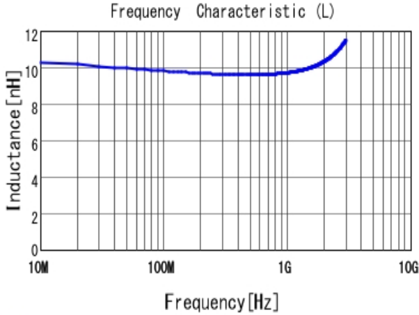
■ LQW15AN10NH00 L
