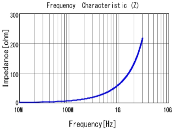
■ LQW15AN10NH00 |Z|
