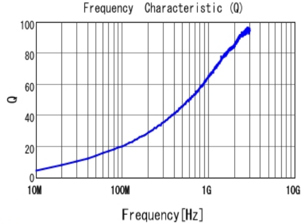
■ LQW15AN10NH00 Q
