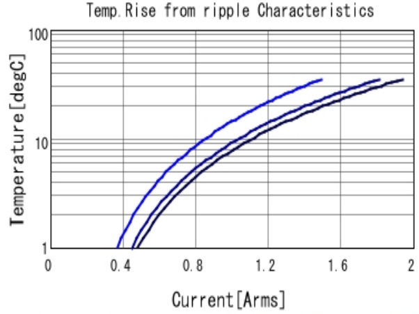
GRM188R61A334KA61 Temp. rise ■ 300kHz ■ 600kHz ■ 1MHz
