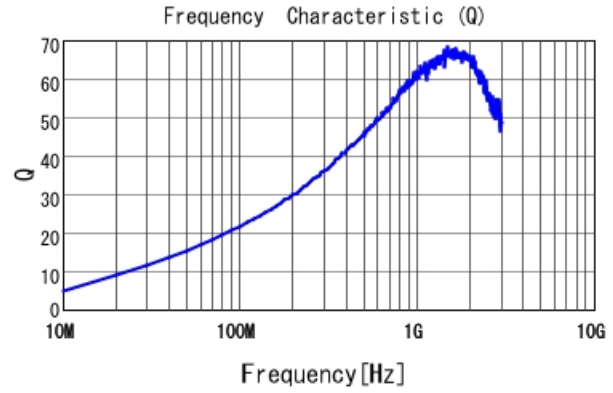
■ LQW15AN40NG00 Q
