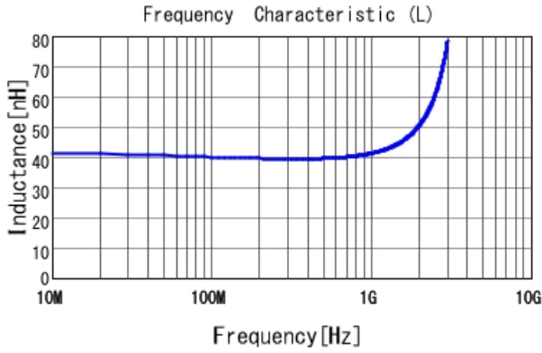
■ LQW15AN40NG00 L
