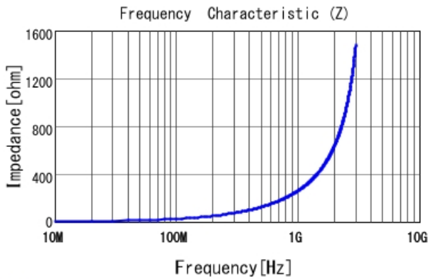
■ LQW15AN40NG00 |Z|
