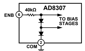
Figure 28. Enable Interface
