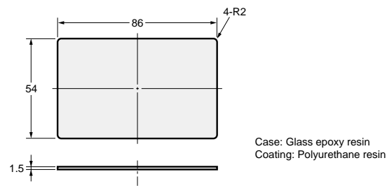
V600-D23P71
