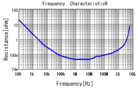
■ GCJ188R71C474KA12 R DCOV, 25degC
