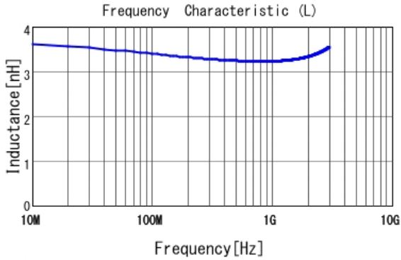
■ LQP03TN3N2B02 L
