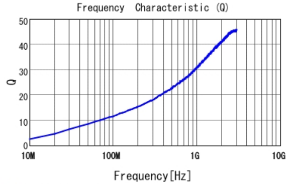
■ LQP03TN3N2B02 Q
