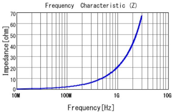
■ LQP03TN3N2B02 |Z|
