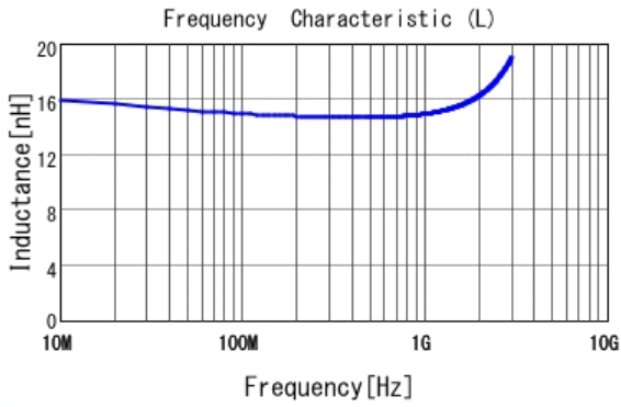
■ LQW15AN15NG00 L
