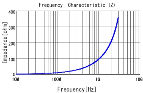
■ LQW15AN15NG00 |Z|
