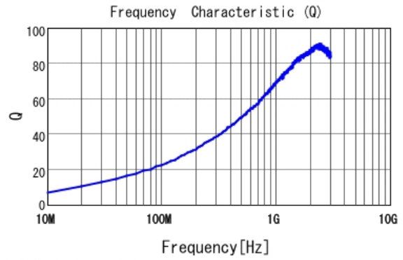
■ LQW15AN15NG00 Q
