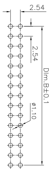
P.C.B Layout
