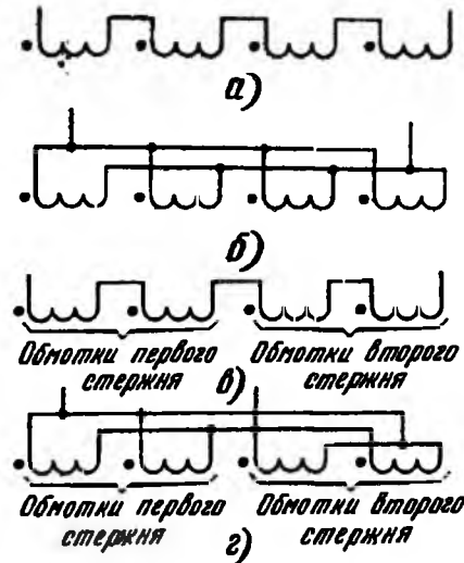
Рис 2.8. Электрические схемы последовательного и параллельного соединений вторичных обмоток трансформаторов типа ТПП: а б — броневой конструкции; в г — стержневой конструкции
