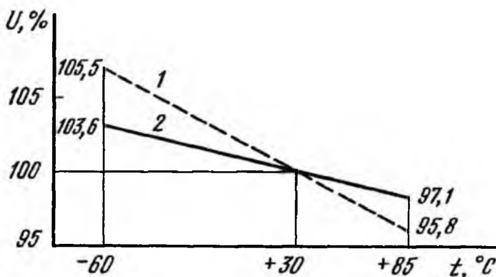
Рис 27 График изменения напряжения вторичных обмоток трансформаторов в режиме номинальной нагрузки в зависимости от температуры окружающей среды 1 — нижний уход напряжения от значения, измеренного при нормальной температуре 2 — средний уход напряжения от значения, измеренного при нормальной температуре
