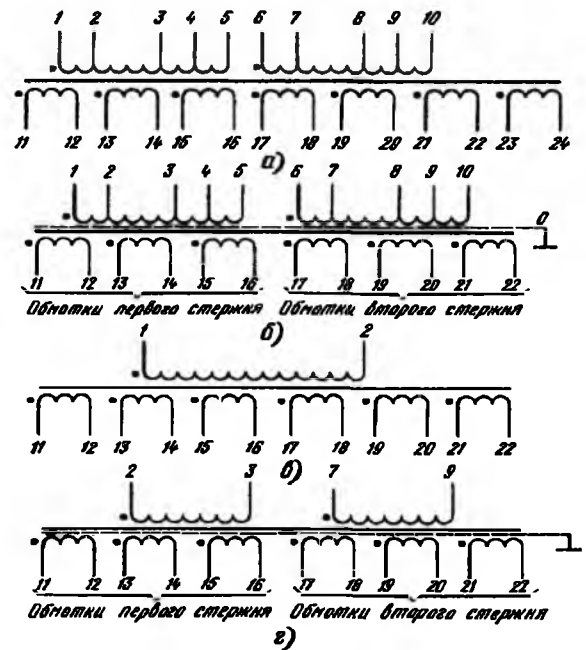
Рис 2.10. Электрические схемы трансформаторов типа ТПП с частотой питающей сети 50 Гц: а — броневой конструкции с напряжением 127/220 В; б — стержневой конструкции с напряжением 127/220 В; в — броневой конструкции с напряжением 220 В; г — стержневой конструкции с напряжением 220 В
