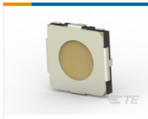
TE Part #2337242-3 TACT MINI JB 5.2X5.2X0.8 260GF
