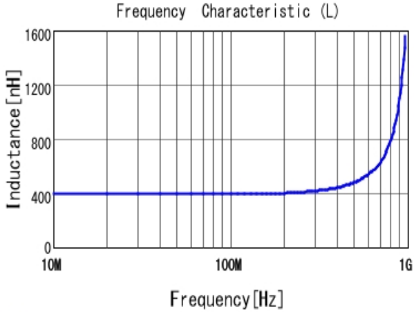
■ LQW18ANR39J00 L
