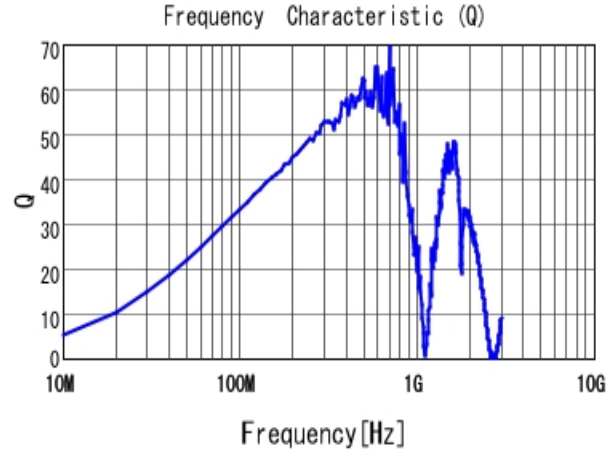
■ LQW18ANR39J00 Q
