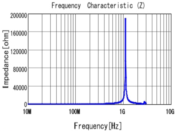
■ LQW18ANR39J00 |Z|
